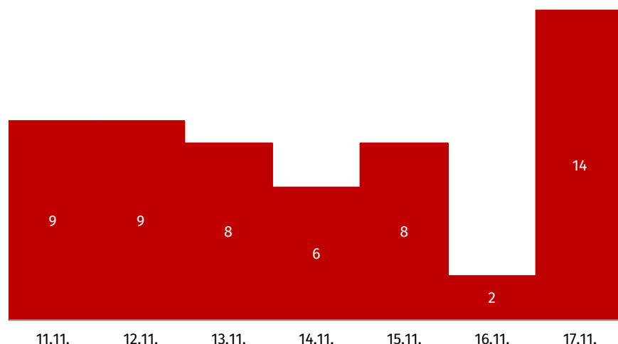
COVID-19-Fälle/ Tag nach Meldedatum
