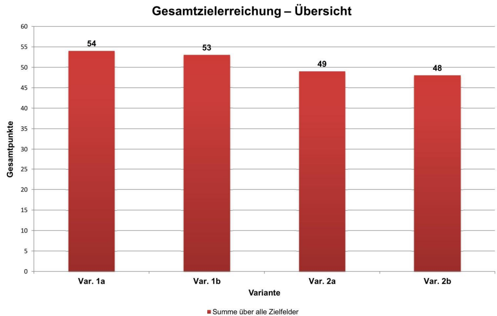
Abb. 56 Gesamtzieelerreichung (Säulendiagramm)
