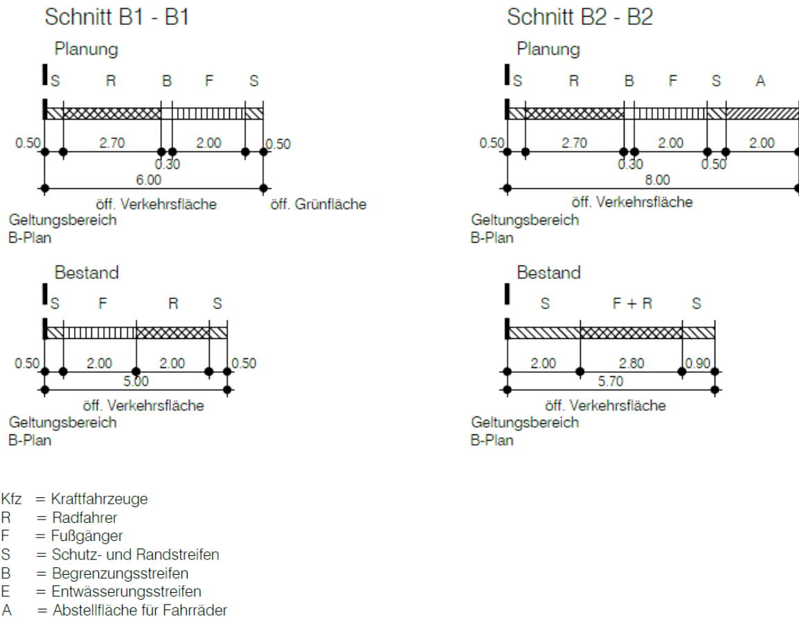
Abb.5: Schnitt B - B
