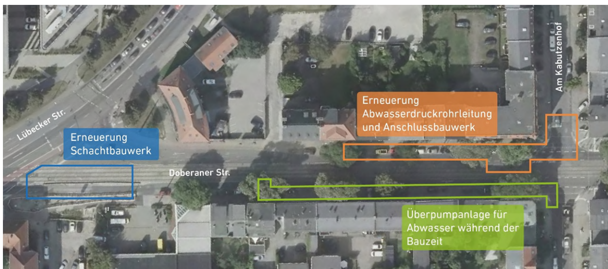
Grafik: Überblick über die einzelnen Baumaßnahmen in Doberaner Straße/Am Kabutzenhof
